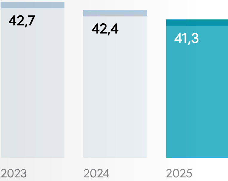
Выбросы парниковых газов, тыс. тон CO 2 -экв
